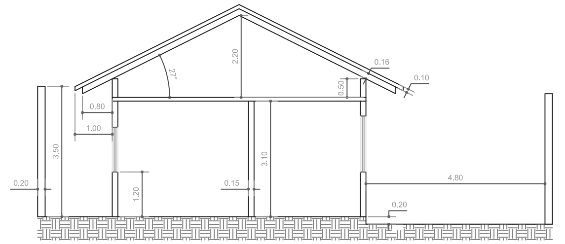
CORTE AA
